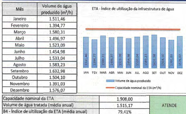
B4 - Índice de utilização da infraestrutura de água (ETA) - Botucatu - Sede
