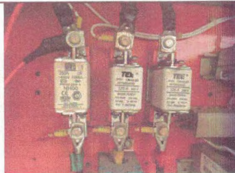
Foto 44 – EEE Jardim Riviera: quadro de comando elétrico - fusíveis com diferentes amperagens.
