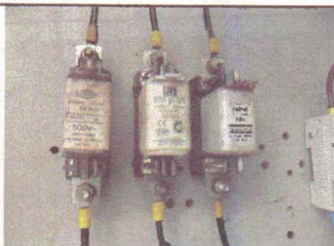
Foto 59 – EEE Jardim Paraíso II: Quadro de comando elétrico - partes vivas expostas.
