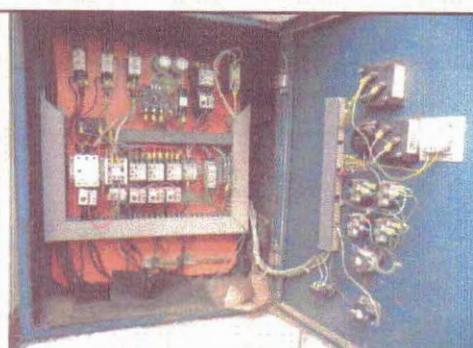
Foto 20 – Quadro de comando elétrico da EEAT: partes expostas.
